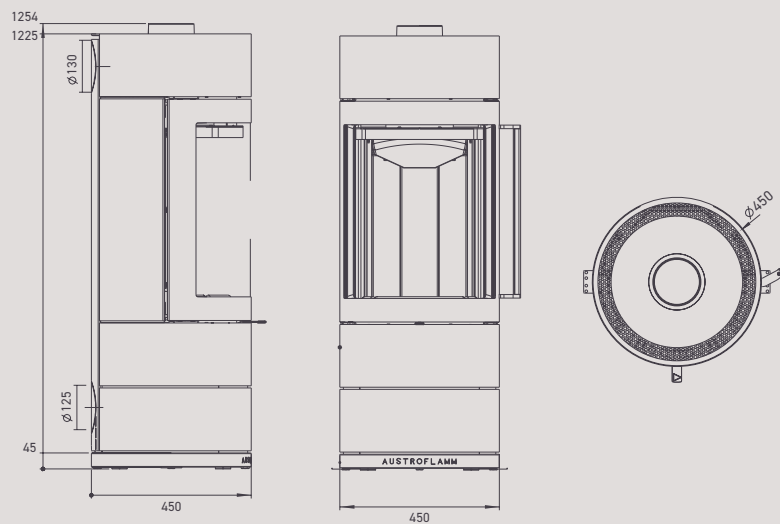
Obr.vlevo: Nyní ještě elegantnější klasika: Lux s horním nástavcem, bočním boxem velkým a dvě dřevěné zásuvky.
