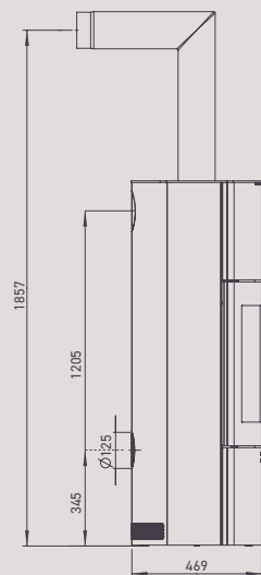
Inovativní: regulovatelná konvekce vzduchu zajišťuje rovnoměrný rozptýl tepla.
