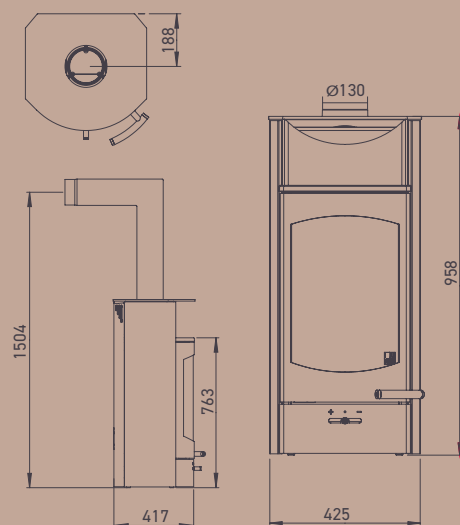
Flok 2.0 s bočním obložním, krytem a nahřívací přihrádkou ze špekového kamene
