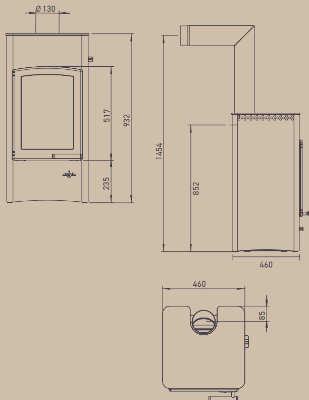
S Lucy Cook můžete vařit, ale nemusíte. I jako tradiční kamna zaujme svým kouzlem.
