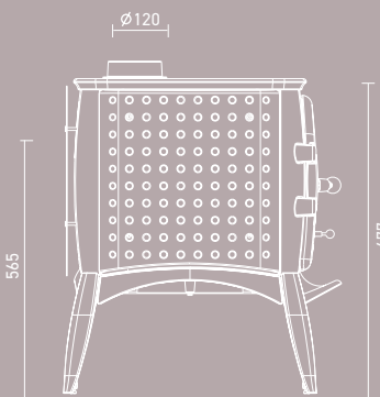
G1 s varnou deskou a konvekčním pláštěm (příslušenství)
