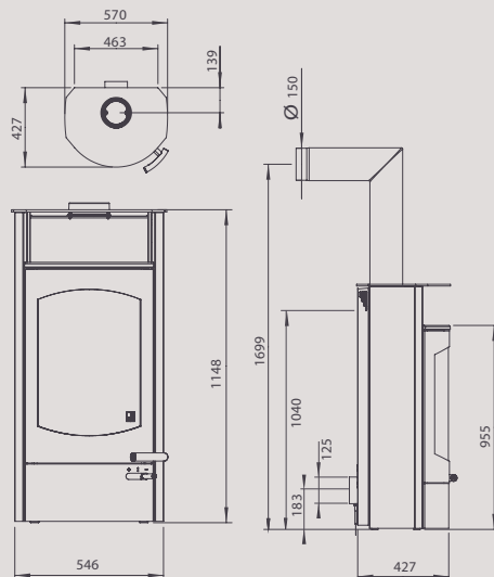
Koko s masťovým obkladem a s ohřívací přihrádkou
