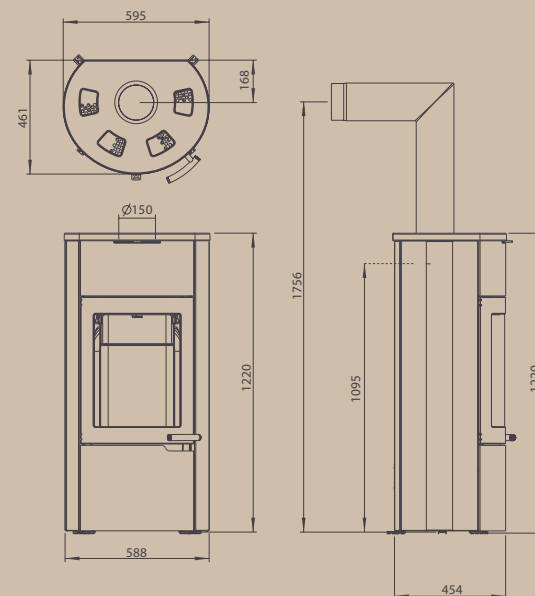
Uno Xtra s obkladem z masťky a horní deskou s nastavitelnými ventilačními otvory.
